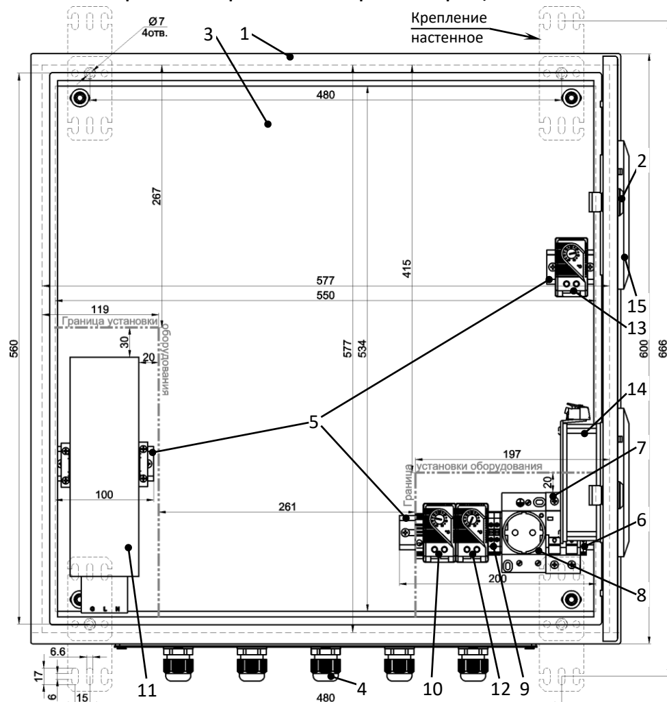
Рисунок 1 – Устройство шкафа
