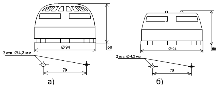
Рисунок 1. Габаритные и установочные размеры извещателей: а) для исполнений ИП212/101-18-R ИБ, ИП212/101-18-А3R ИБ; б) для исполнений ИП212/101-18-А1 ИБ, ИП212-18 ИБ.
