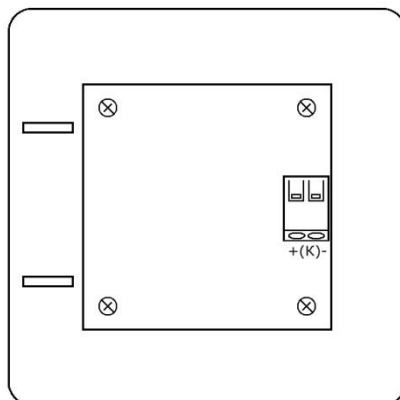
Рисунок 2. Внешний вид платы кнопки сброса вызова GC-0421W1
